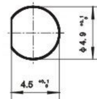
安装开孔尺寸 Mounting hole
