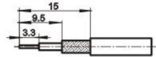
电缆剥线尺寸 Cable stripping dimensions
