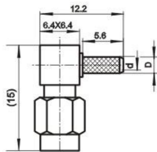
电缆剥线尺寸 Cable stripping dimensions
