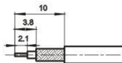
电缆剥线尺寸 Cable stripping dimensions
